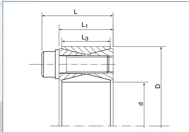
Spansatz / Locking Assembly RfN 7012 · Maßzeichnung / Dimensions
